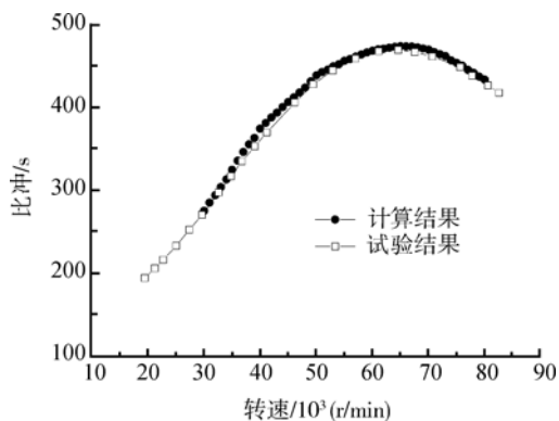
图7 比冲与转速的关系
