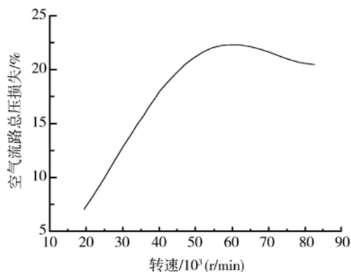
图 3 空气流路总压损失与转速的关系
