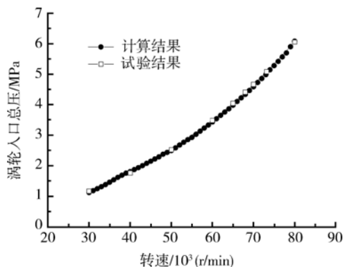
图 9 涡轮入口总压与转速的关系
