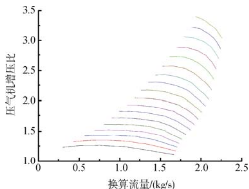
图 2 压气机特性
