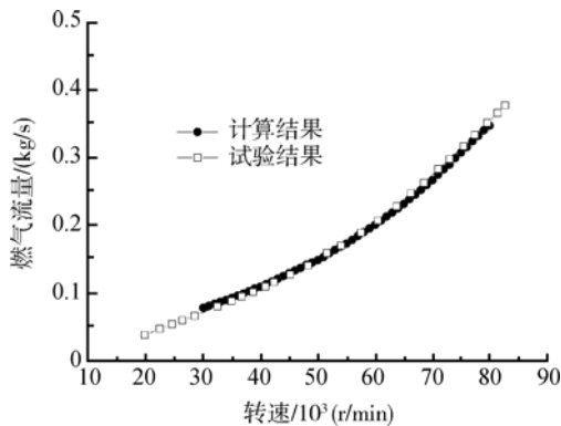
图5 燃气流量与转速的关系
