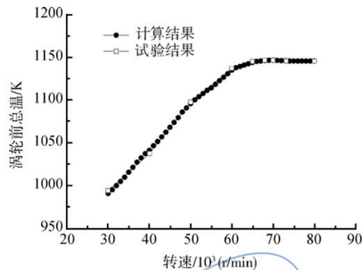
图 10 涡轮前总温与转速的关系
