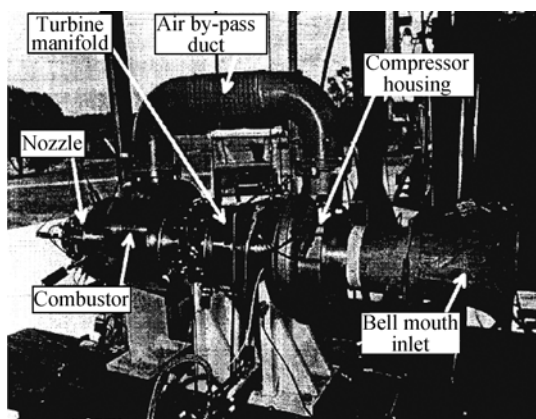
图 1 ATR 结构图
