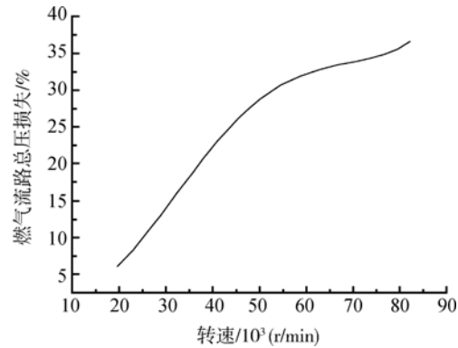
图 4 燃气流路总压损失与转速的关系
