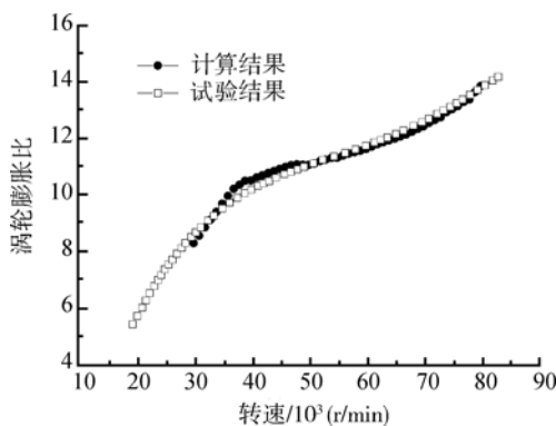
图 8 涡轮膨胀比与转速的关系
