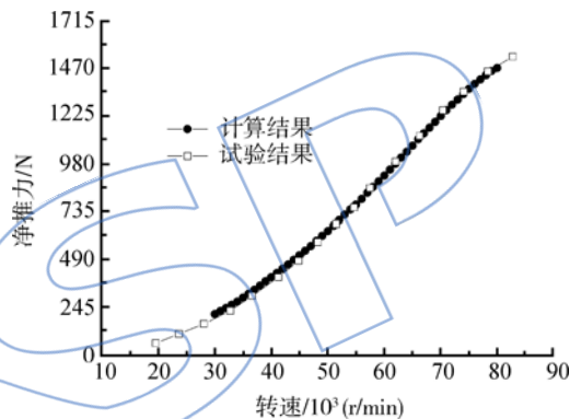
图6 净推力与转速的关系
